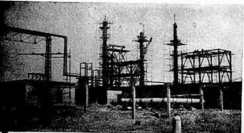
بوسكام نېفىت - خىمىيە سانائىتىنى زاۋۇتىنىڭ ئىش ئورنىدىن چىقىرىۋېتىش شىۋى ئوتتۇرىسى .
